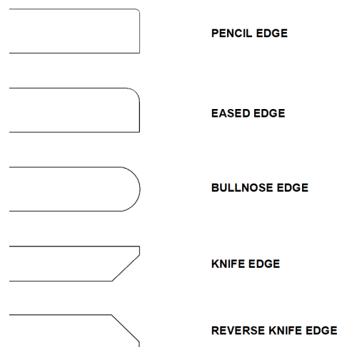
Edge Profiles
